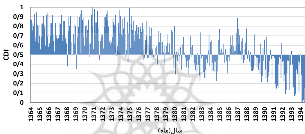
شکل ۸: سری زمانی شاخص CDI در پیژومتر شماره ۲۰ در دشت شهرکرد (۱۳۶۴ تا ۱۳۹۴)
