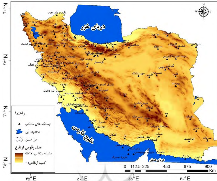
شکل ۱: ایستگاه‌های همدید مورد مطالعه
