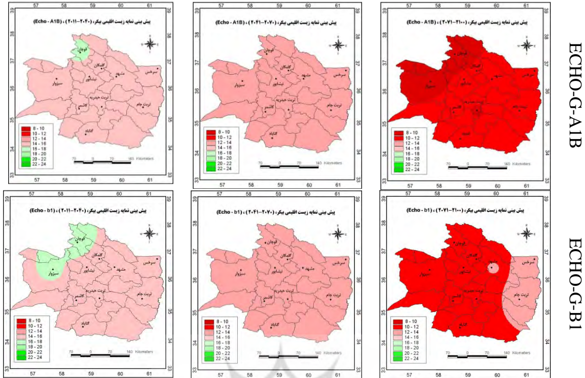
شکل (۵) شبیه سازی نمایه بیکر در استان خراسان رضوی برای دوره ۲۰۱۱-۲۱۰۰ با استفاده از مدل گردش
