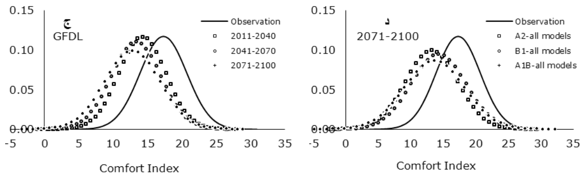
شکل (۷) شبه سازی تابع چگالی نمایه زیست اقلیم بیکر در استان خراسان رضوی توسط مدل های الف- CGCM، ب- ECHO-G، ج- GFDL در دوره های مختلف و د- تمامی مدل ها در دوره ۲۰۷۱-۲۱۰۰ تحت سناریوهای انتشار مختلف.
