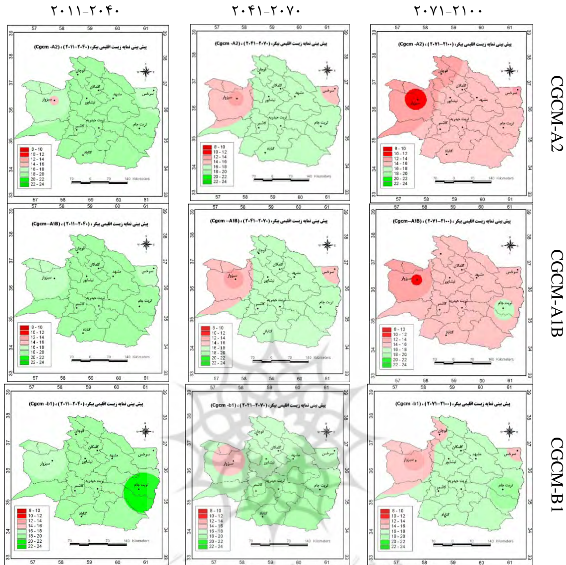
شکل (۴) شبیه سازی نمایه بیکر در استان خراسان رضوی برای دوره ۲۰۱۱-۲۱۰۰ با استفاده از مدل گردش عمومی تحت سه سناریوی انتشار A2، A1B و B1
