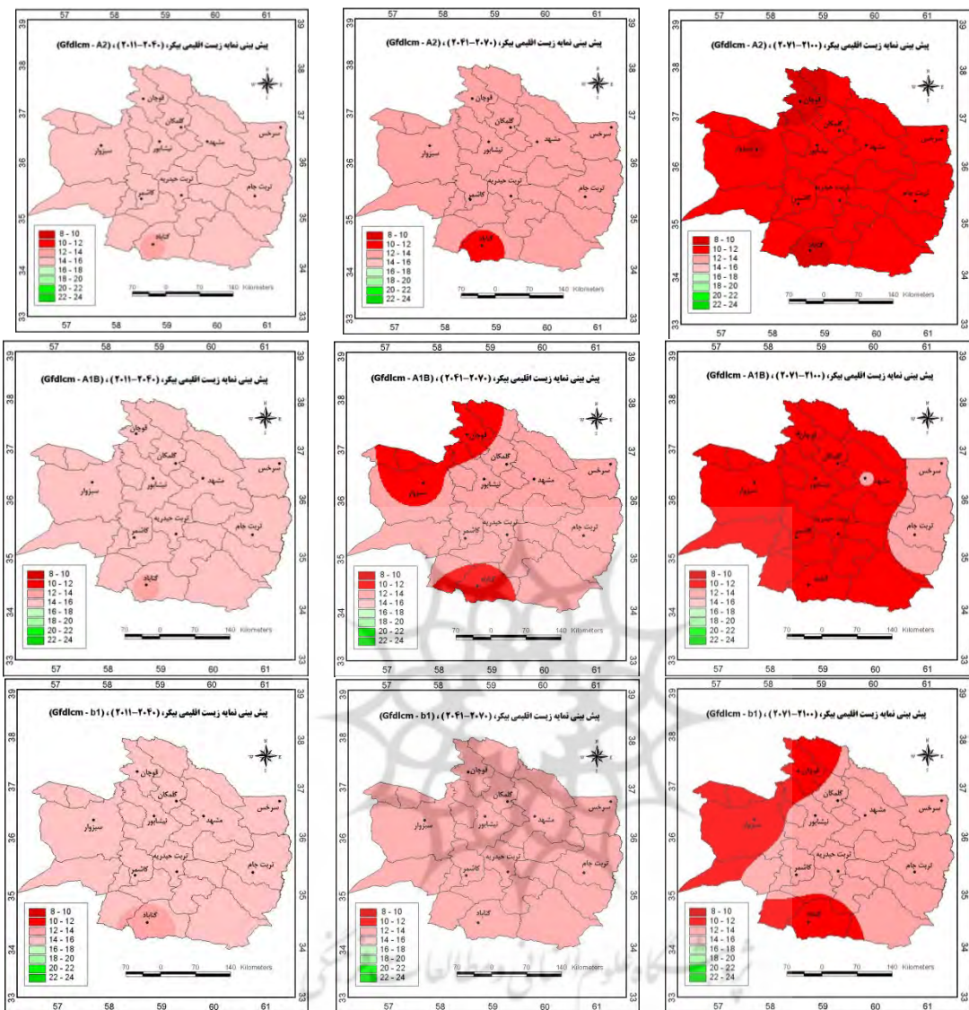
شکل (۶) شبیه سازی نمایه بیکر در استان خراسان رضوی برای دوره ۲۰۱۱-۲۱۰۰ با استفاده از مدل گردش عمومی
