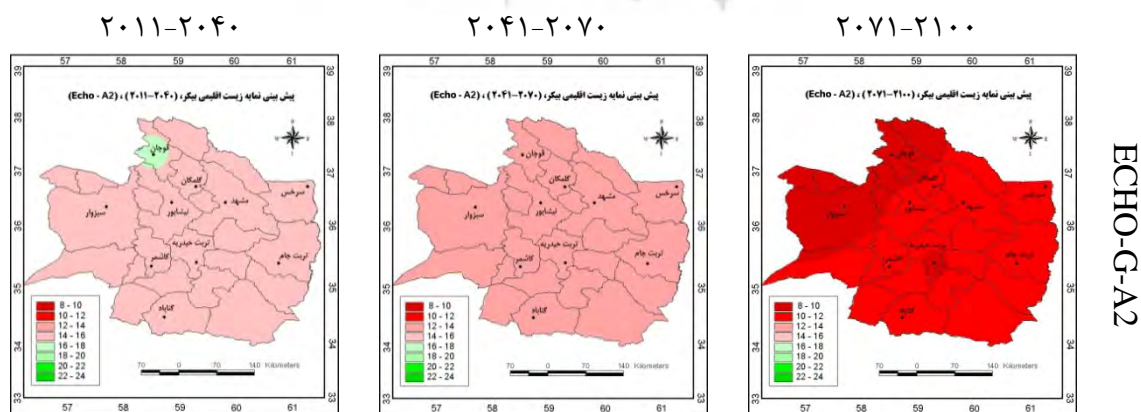
شکل (۴) شبیه سازی نمایه بیکر در استان خراسان رضوی برای دوره ۲۰۱۱-۲۱۰۰ با استفاده از مدل گردش عمومی تحت سه سناریوی انتشار A2، A1B و B1
