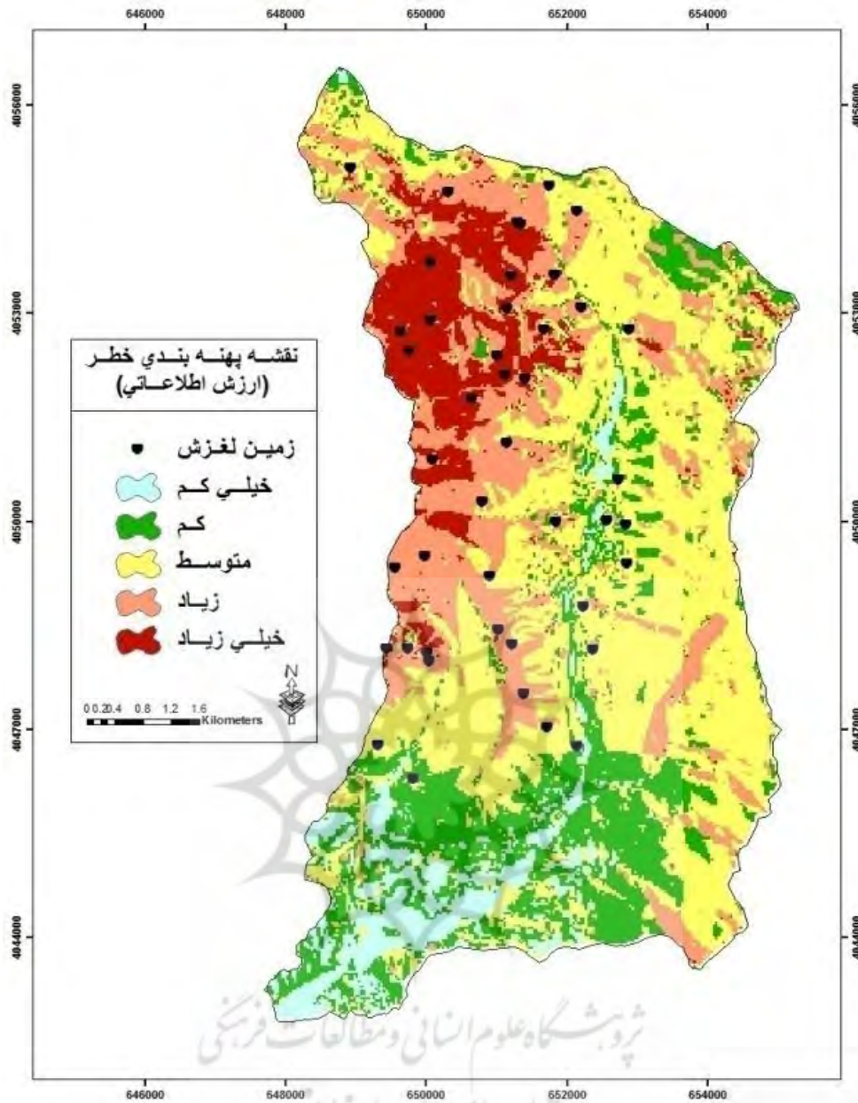
شکل (۱۴): نقشه‌ی پهنه‌بندی خطر زمین‌لغزش به روش LNRN
