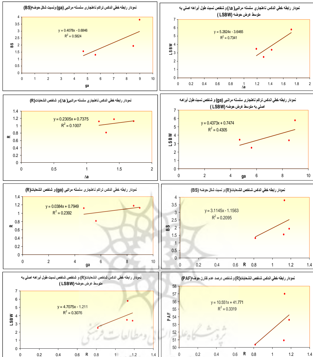
شکل ۴: رابطه خطی و مقدار ضریب تبیین بین ga ، \Delta a و R و پارامترهای BS ، LSBW ، PAF در حوضه‌های مورد مطالعه (منبع: نگارندگان)
