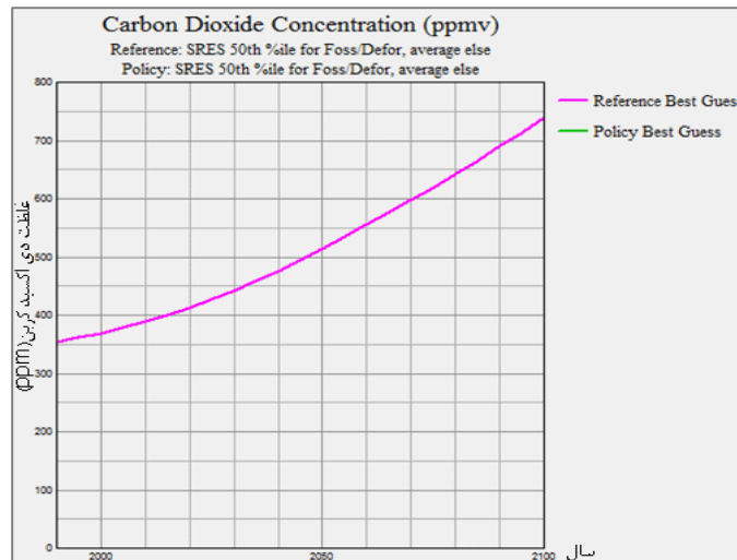
شکل ۱. نحوه انتشار دی اکسید کربن به‌وسیله سناریوی بدبینانه P50
