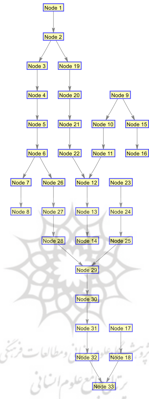
شکل (۱۳): توپولوژی شبکه ۳۳ باس در حالت اول
