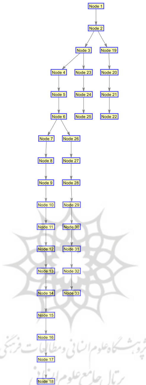
شکل (۱۶): توپولوژی شبکه ۳۳ باس در حالت چهارم
