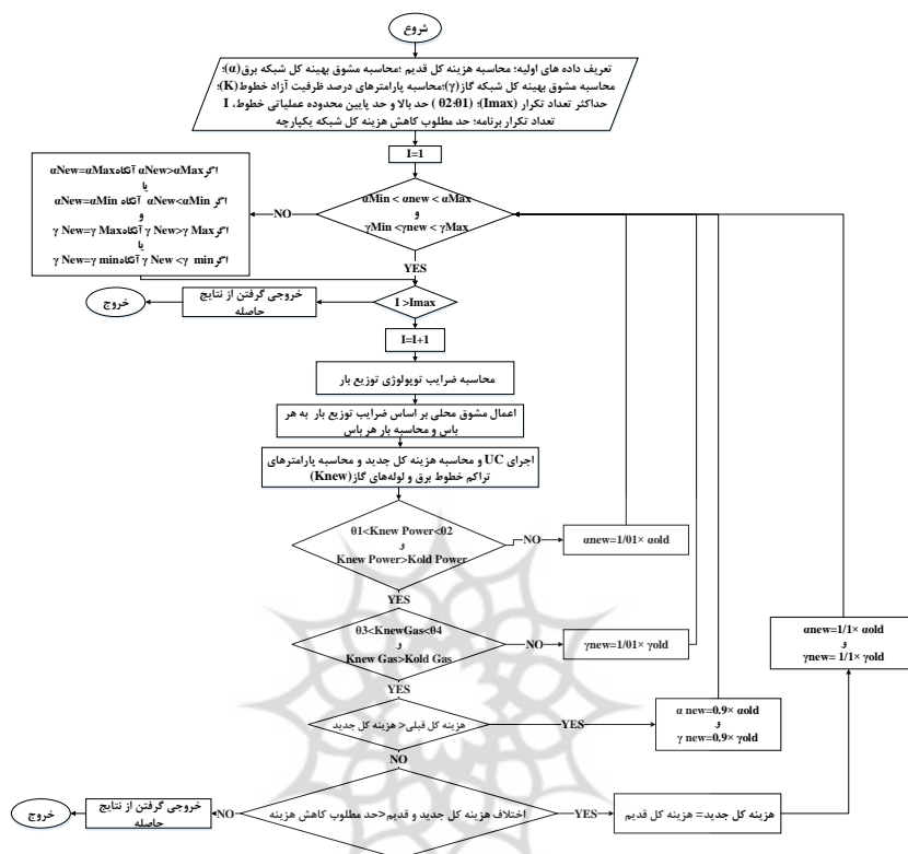
شکل ۱. فلوجارت حل مسئله‌ی تلفیقی در شبکه برق و گاز
