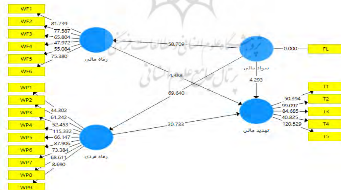
شکل (۱): مدل اصلی در حالت اعداد معناداری (t_value)
