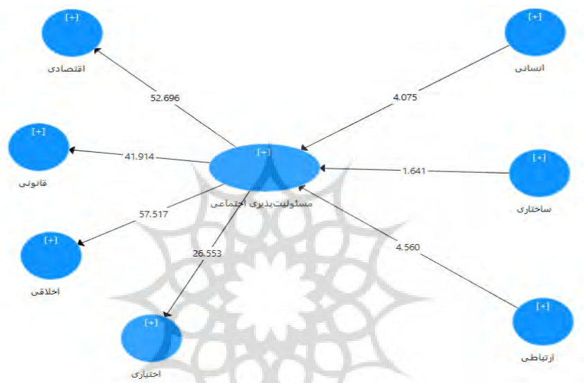
شکل ۳. مدل ضرایب معناداری پژوهش - مدل فرعی
