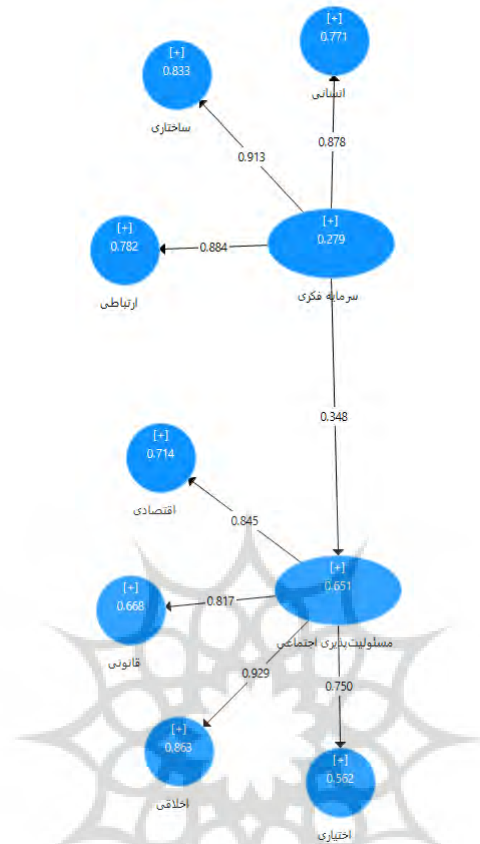
شکل ۲. مدل ضرایب استاندارد - مدل اصلی
