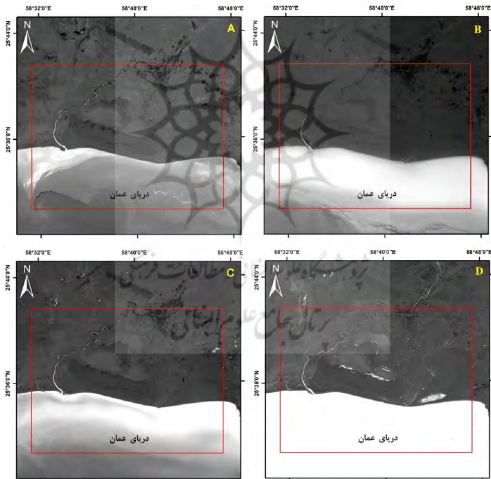
شکل ۳. شاخص طیفی NDWI دلتای سدیج در سال (A: ۱۳۹۲ B: ۱۳۹۵ C: ۱۳۹۷ D: ۱۳۹۸)
