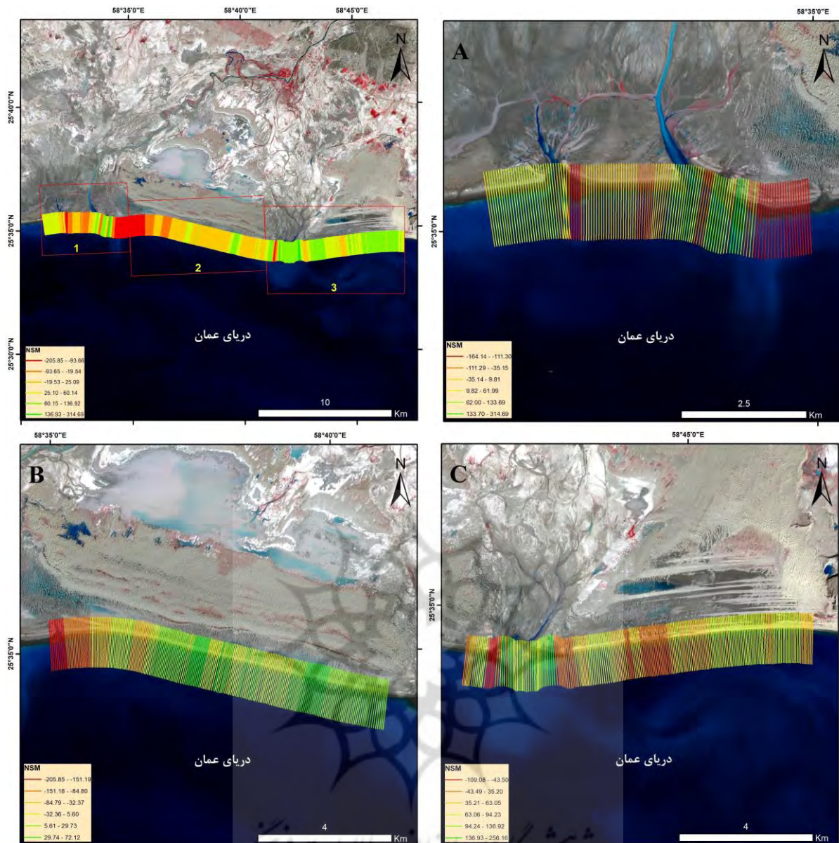
شکل ۷ تغییرات خطوط ساحلی بر مبنای ترانسکت شاخص NSM برای ۴ سیلاب (بر روی تصویر لندست ۲، سال ۲۰۲۰): A: بازه ۲، B: بازه ۱، C: بازه ۲، D: بازه ۳
