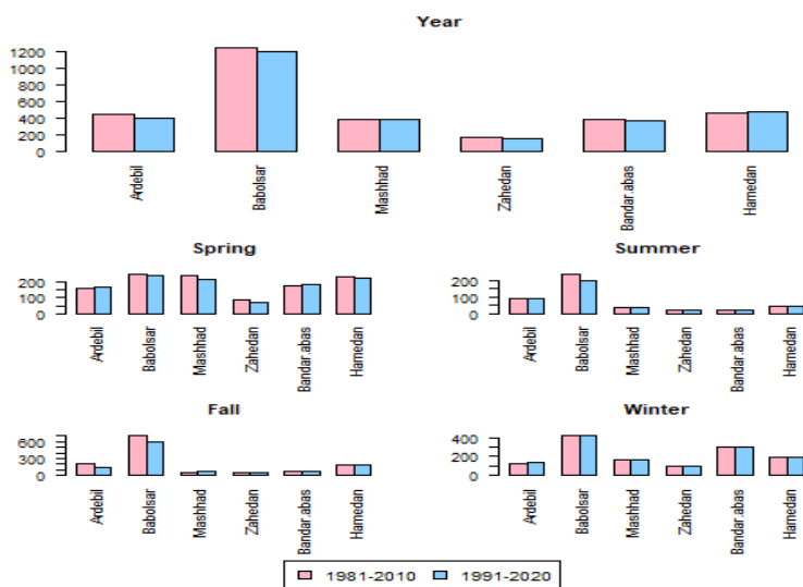
شکل ۲- چندک ۰/۹۸ بارش سالانه و فصلی برای ایستگاه‌های منتخب
