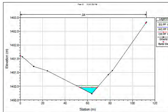
شکل ۱۷: مقطع عرضی حداکثر ارتفاع سطح آب با دوره‌ی بازگشت ۲۵ ساله برای حوضه B، منبع: نویسندگان، ۱۴۰۲.
