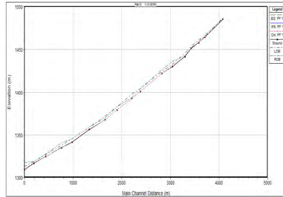
شکل ۱۰: پروفیل طولی حوضه A برای سیل با دوره ۱۰ سال در حداکثر ارتفاع سطح آب، منبع: نویسندگان، ۱۴۰۲.
