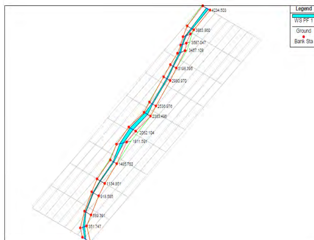
شکل ۱۴: نمای ۳ بعدی از سطوح سیلاب گیر در طول رودخانه به ازای دوره بازگشت ۲۵ ساله، منبع: نویسندگان، ۱۴۰۲.
