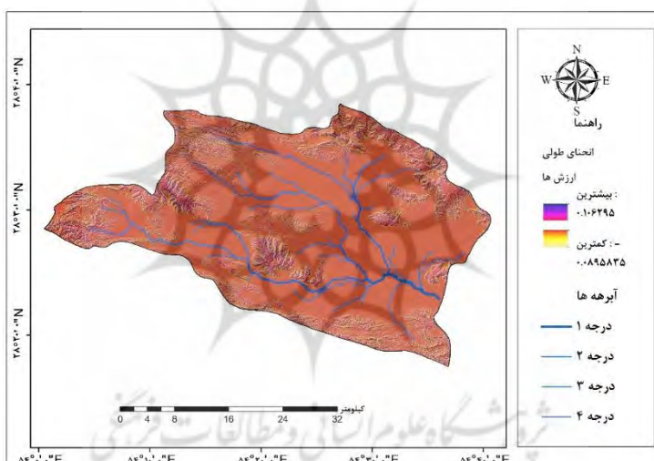
شکل ۷: نقشه انحنای طولی حوضه آبخیز خسویه
