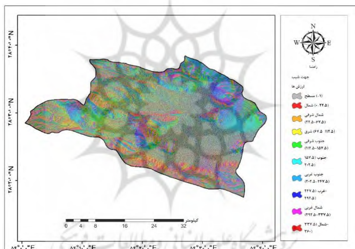
شکل ۴: نقشه جهت شیب حوزه آبخیز خسویه
