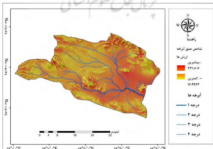
شکل ۵: نقشه عمق آبراهه حوزه آبخیز خسویه
