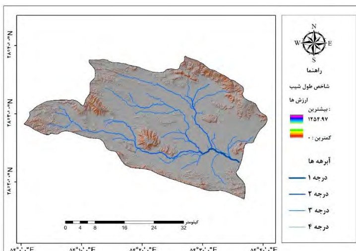
شکل ۶: نقشه طول شیب حوضه آبخیز خسویه
