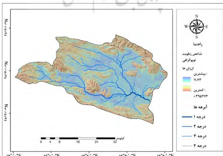
شکل ۸: نقشه رطوبت توپوگرافی حوضه آبخیز خسویه
