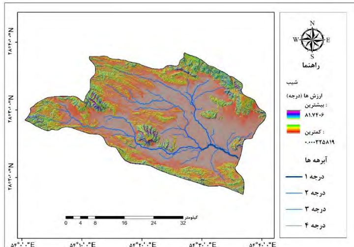
شکل ۳: نقشه شیب حوزه آبخیز خسویه
