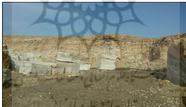
شکل ۶- متروکه شدن معدن به دلیل توسعه شکستگی‌های کششی و برشی، جهت دید (NE)
