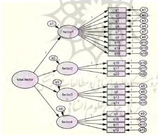
نمودار ۱: دیاگرام تحلیل عاملی تائیدی برازش شده مرتبه دو نمایه‌سازی تصاویر در موتورهای جستجو در بازیابی تصاویر نمایه شده مبتنی بر متن و محتوا
