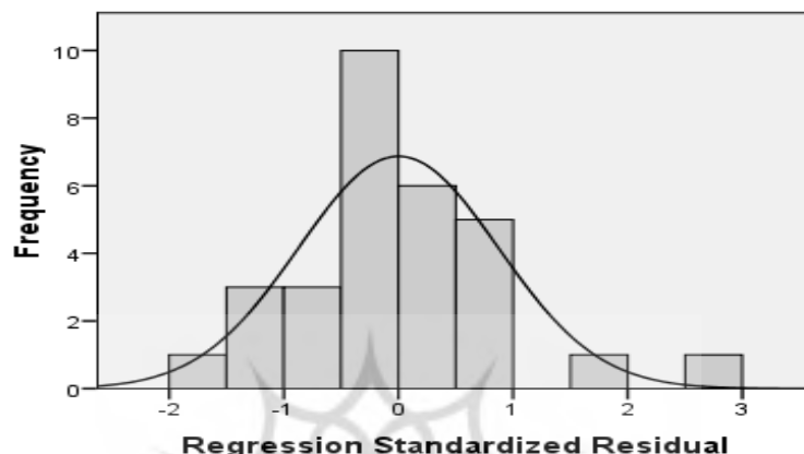
نمودار ۲. هیستوگرام مربوط به مانده‌ها در برازش مدل رگرسیونی
