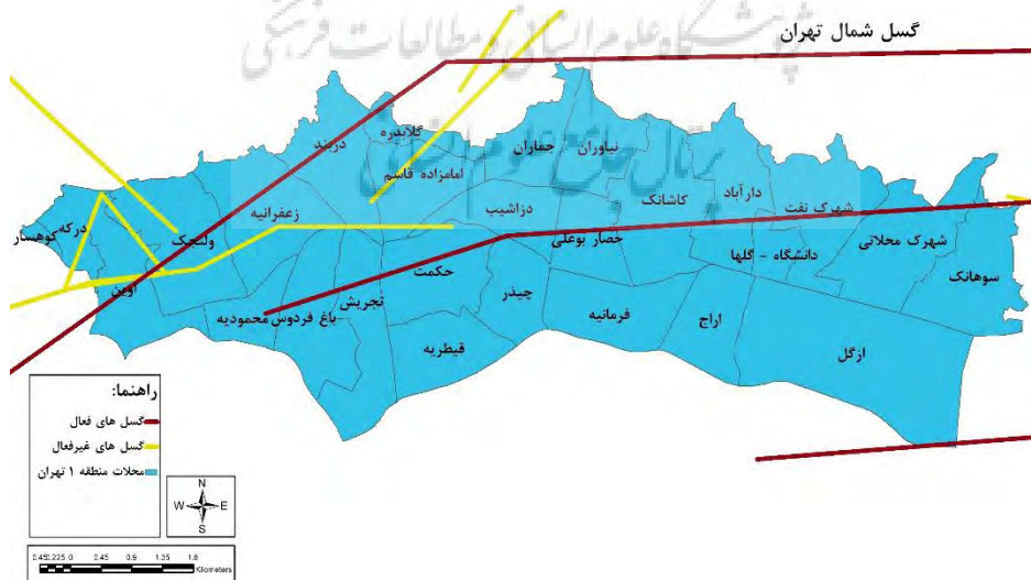
تصویر ۳- نقشه گسل های فعال و غیرفعال منطقه ۱ شهرداری تهران
