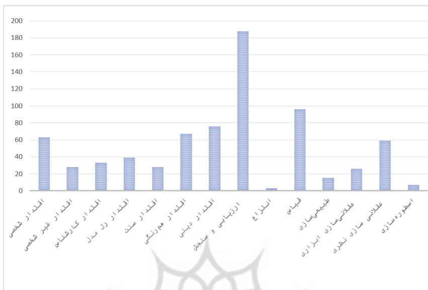
نمودار ۱. بسامد مؤلفه‌های مشروعیت‌بخشی در امثال
