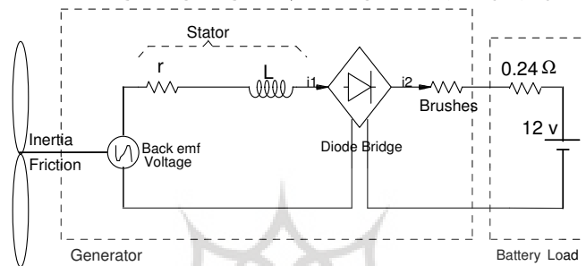
شکل ۱۰: مدل الکتریکی
