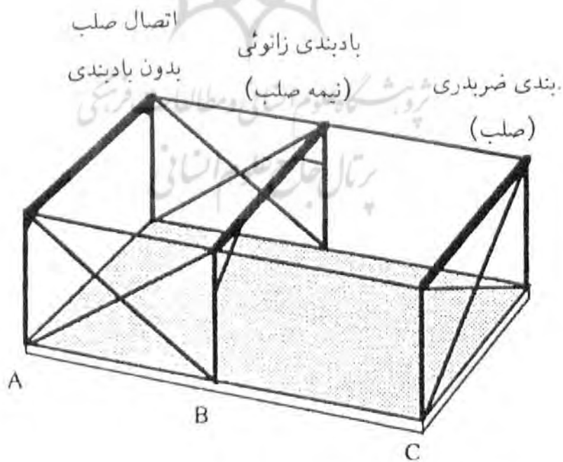
شکل ۵. مدلی با سه قاب پرتابیل با سختی مختلف در هر صفحه
