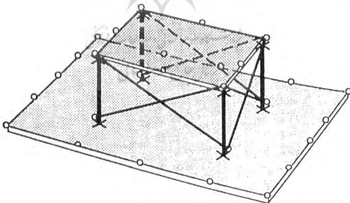
شکل ۴. سه دیوار برشی که به صورت ضربدری مهاربندی شده‌اند
