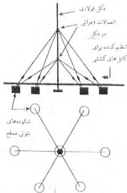
شکل ۷. دکل با مهاربندی
