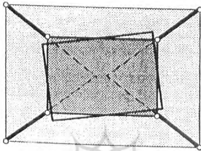
شکل ۶. پلان شکل ۱ یا مهار گوشه که نشان‌دهنده ساختار بد مهاربندی است
