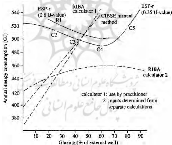
شکل ۵: پیش‌بینی انرژی مصرفی با استفاده از روش‌ها و پیشفرض‌های مختلف (Clarke, 2001)
