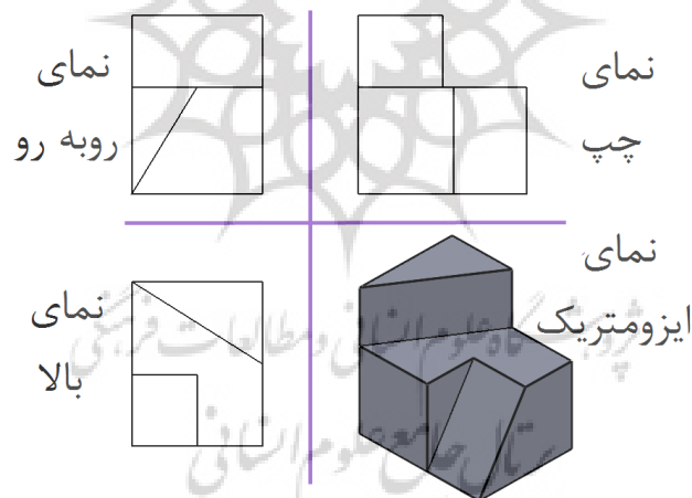
شکل ۱: نمونه‌ای از یک نقشه استاندارد
