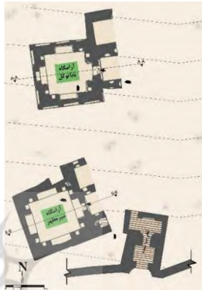
تصویر ۱۲: پلان آرامگاه باباتوکل و آرامگاه میرمطهر
