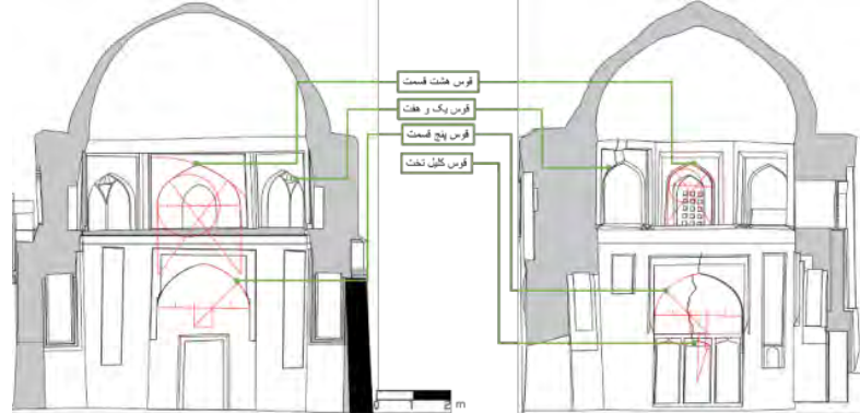
تصویر ۲۴: قوس‌های پنج قسمت و هشت قسمت در آرامگاه‌های باباتوکل (سمت راست) و میرمطهر (سمت چپ) و قوس کلیل تخت در آرامگاه باباتوکل.
