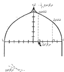
تصویر ۵۲: نحوه ترسیم چفد سه‌قوسی. (مأخذ: رئیس‌زاده و مفید، ۱۳۸۹: ۱۸).
