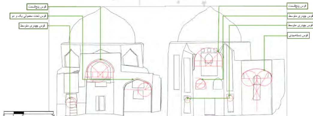
تصویر ۲۳: نوع چفدها به ترتیب از سمت راست به چپ: دسته‌سبیدی، پنج قسمت، چیدری متوسط، تخت معمولی یک و دو، پنج قسمت.
