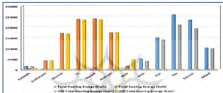
شکل ۲۸: مقایسه مصرف انرژی در حالت ساده و با نمای دوپوسته ۸۰ سانتی متری (مأخذ: نگارنده)
