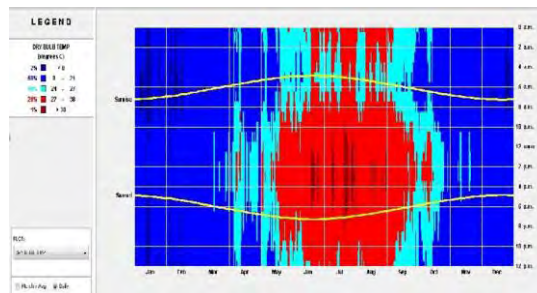
شکل ۲: جدول زمانی دما برای ماه‌های مختلف (مأخذ: نگارنده)
