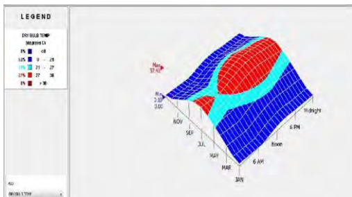
شکل ۳: طرح ۳ بعدی دما برای ماه و ساعت مختلف (مأخذ: نگارنده)
