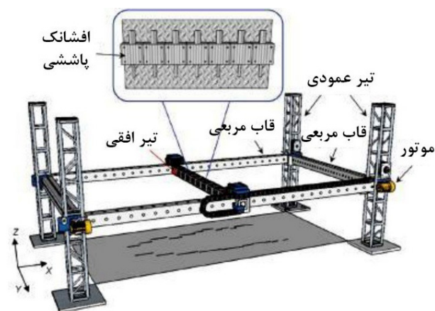
تصویر ۳. چاپگر D-Shape. مأخذ: Al-Safy, 2019.
