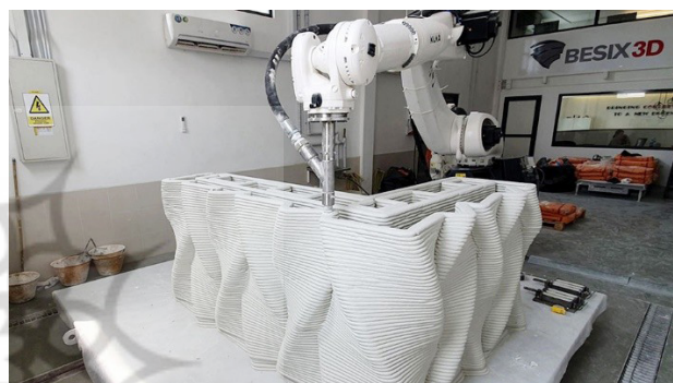
تصویر ۴. چاپ سه‌بعدی بتن. مأخذ: www.kuka.com.
