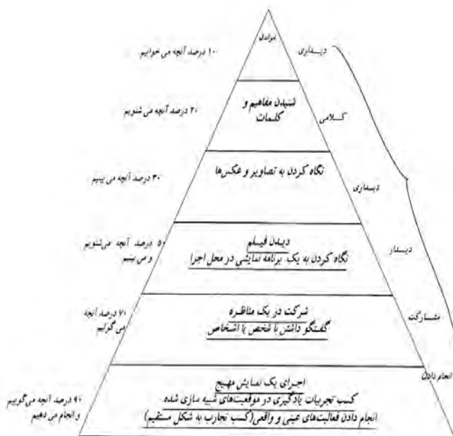
شکل ۱- مخروط یادگیری
