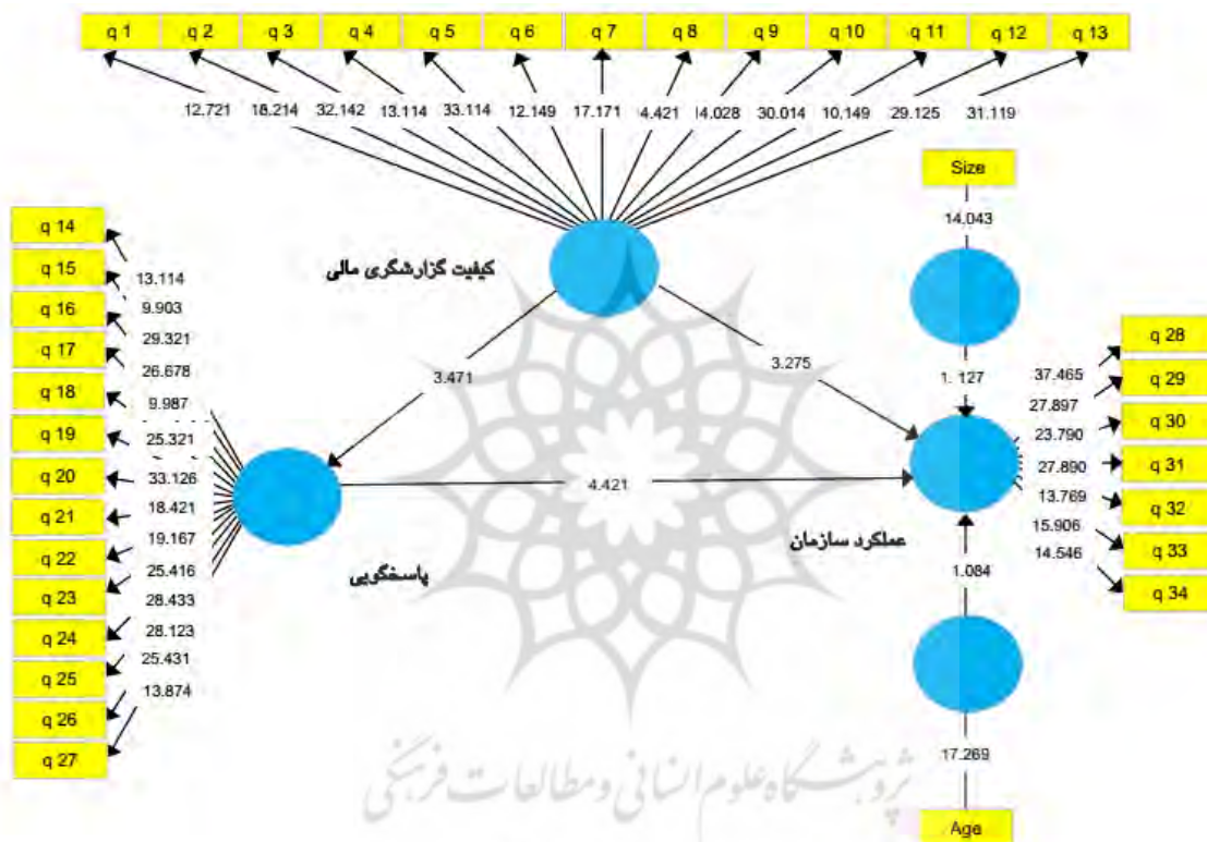
شکل (۱): مدل معادلات ساختاری تحقیق در حالت معناداری
