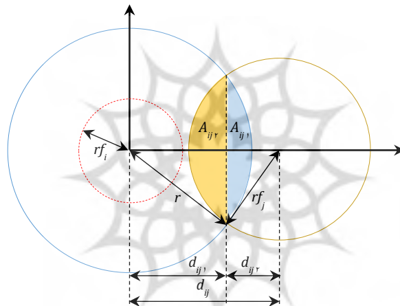
شکل ۳. سطح همپوشانی بین دو نقطه مجاور
