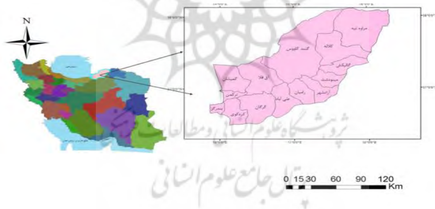
شکل ۱ - نقشه استان گلستان و شهرستان‌های تابعه آن (منطقه مورد مطالعه)
