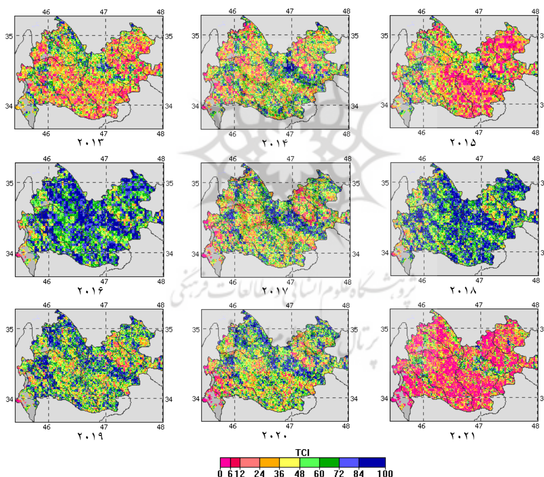
شکل ۲. میانگین هفتگی Temperature Condition index (TCI) استان کرمانشاه (هفته ۲۶) اول جولای (۲۰۲۱-۲۰۱۳)،
