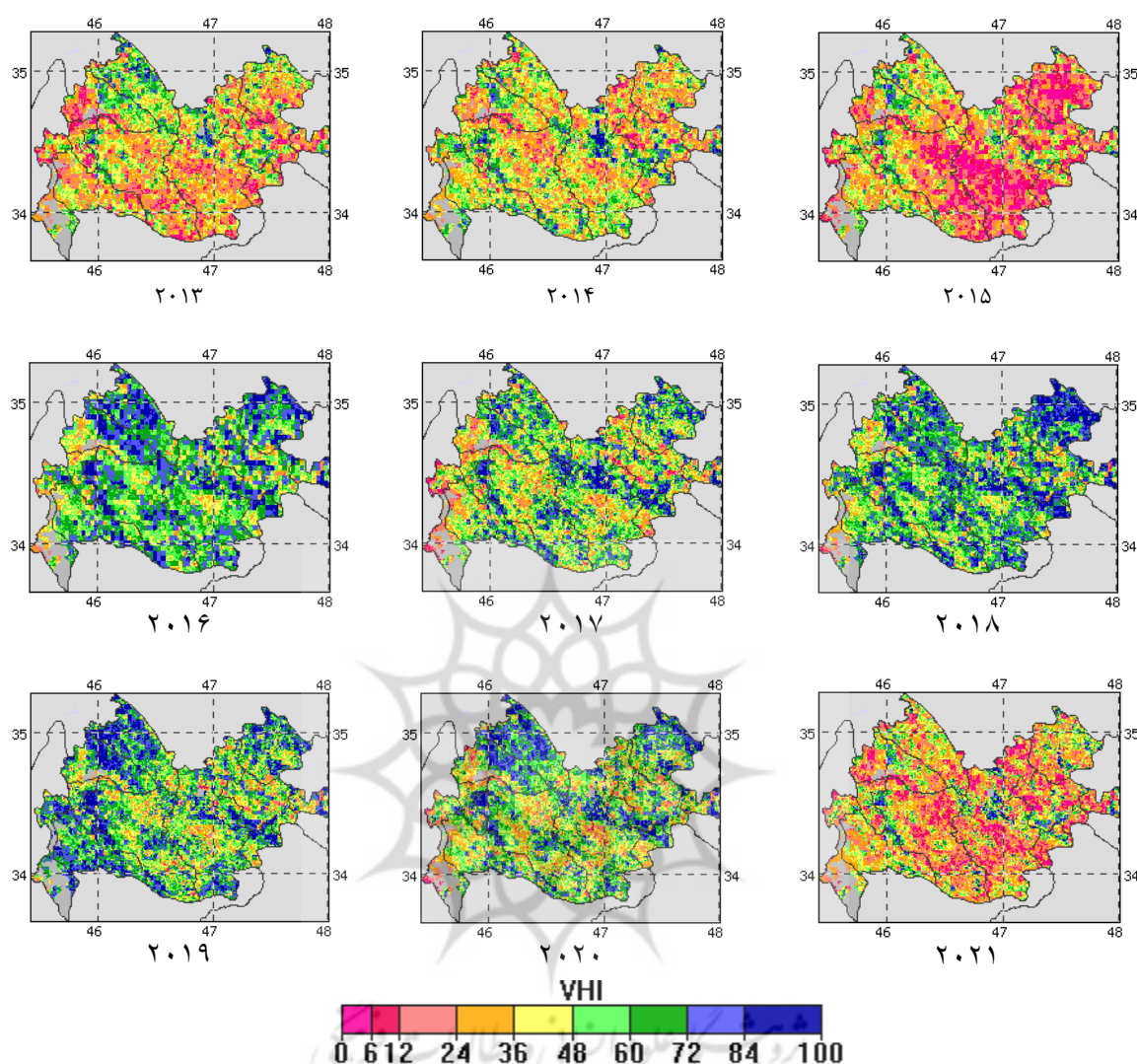
شکل ۴. میانگین هفتگی Vegetation Health index (VHI) استان کرمانشاه (هفته ۲۶) اول جولای (۲۰۱۳-۲۰۲۱)، منبع: نگارندگان، ۱۴۰۱ با توجه به شکل (۴) ملاحظه می‌شود که در منطقه مورد
