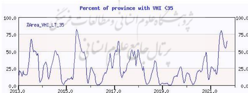
شکل ۱۳. میانگین هفتگی شاخص سلامت گیاهی سری زمانی <35 (VHI) استان کرمانشاه، منبع: نگارندگان، ۱۴۰۱
