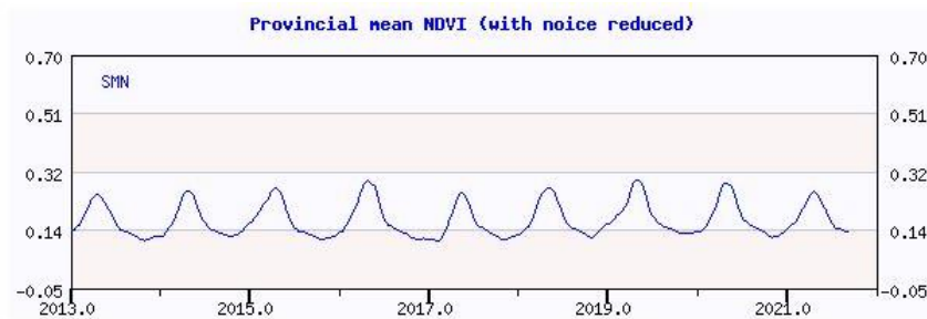
شکل ۸. میانگین هفتگی سری زمانی میانگین هفتگی استانی NDVI استان کرمانشاه، منبع: نگارندگان، ۱۴۰۱
