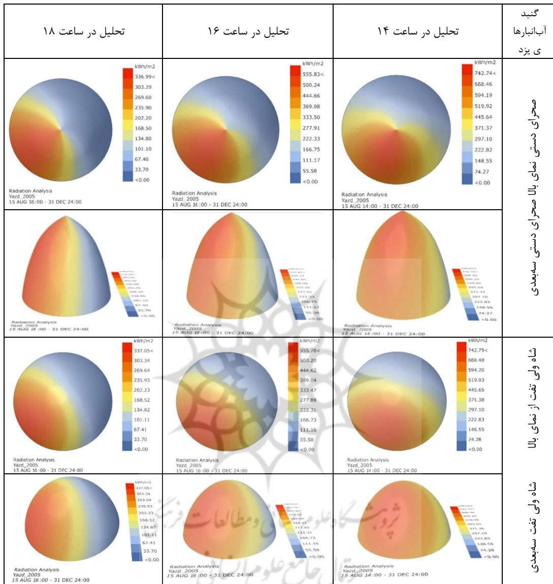
شکل (۵). تحلیل دریافت تابش خورشیدی، جذب حرارت در محدوده سایه بر سطوح گنبد آب‌انبارهای یزد بر حسب kwh/m^2 . منبع: انرژی پلاس (هانی بی و لیدی باگ) منبع: نگارندگان.
