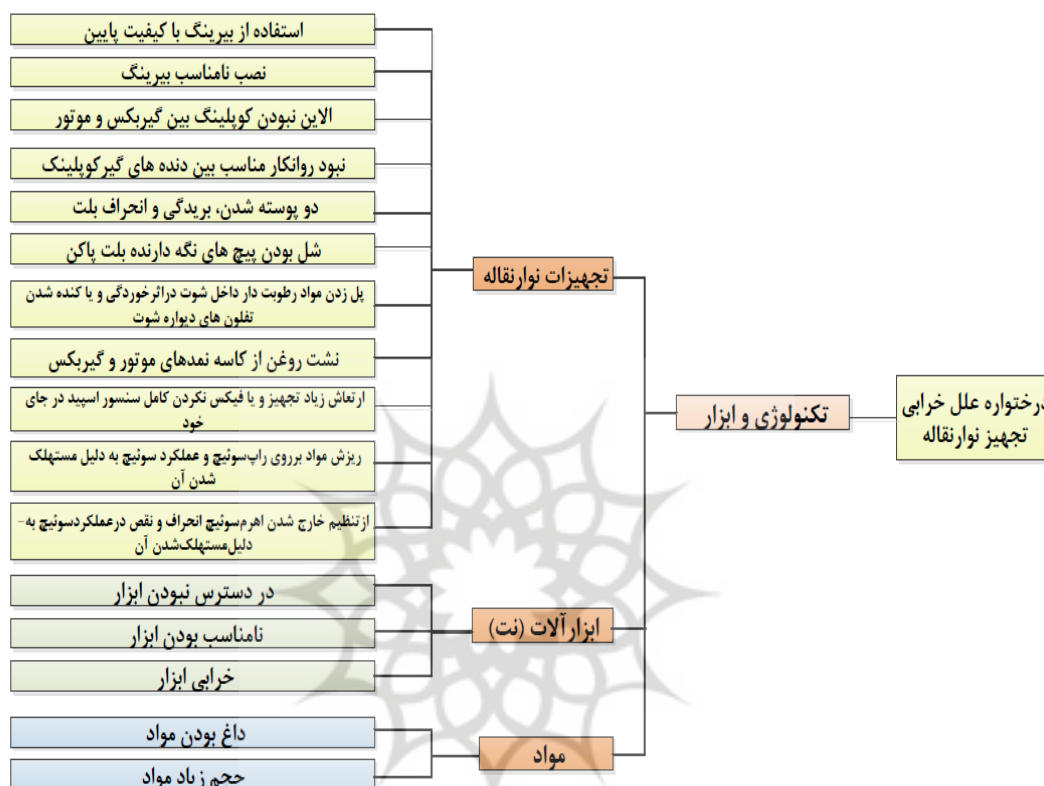
شكل ۱: درختواره علل خرابى تجهيز نوار نقاله
