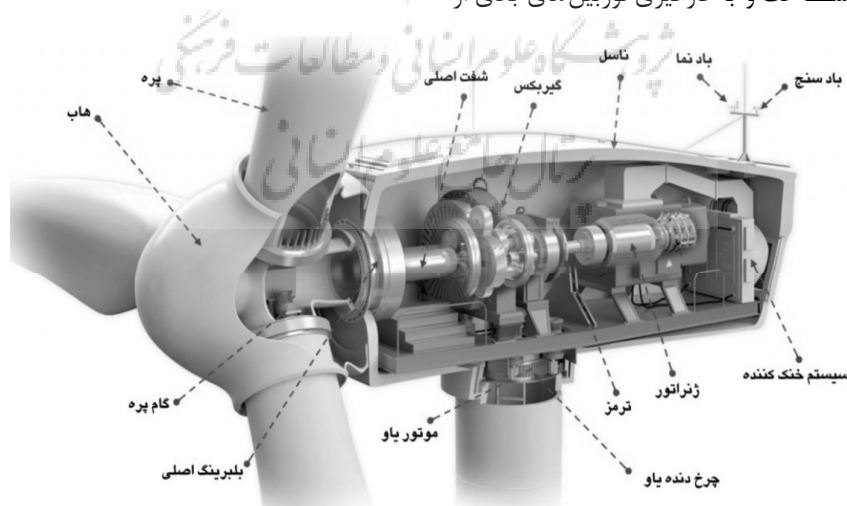
شکل ۱- شمای کلی از قطعات اصلی یک توربین بادی
