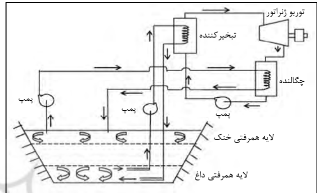
شکل 21: چرخه تولید الکتریسیته از حوضچه خورشیدی
