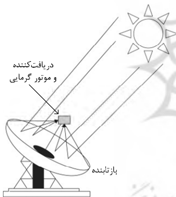
شکل 18: طرحواره یک بشقاب خورشیدی
