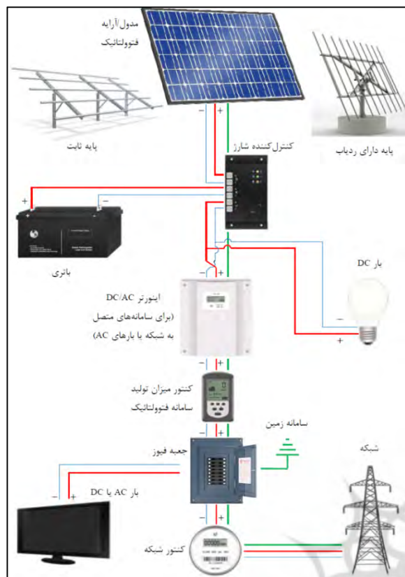
شکل 3: فرآیند تولید انرژی الکتریکی در سامانه‌های فتوولتائیک
