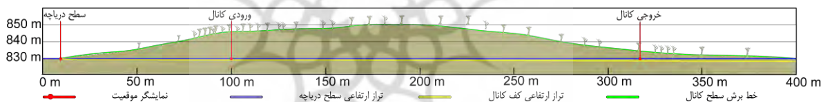
شکل ۱: نقشه پروفیل طولی (شمال غرب به جنوب شرق) کانال پل نگین (Sadeghirad, 2016: 65)
