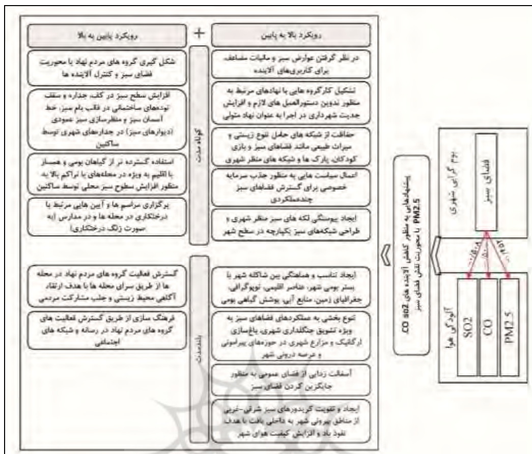
شکل ۱۴. پیشنهادهایی به منظور کاهش آلاینده‌های CO, SO 2 و PM 2.5 با محوریت نقش فضای سبز
