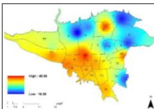
شکل ۱۰. وضعیت غلظت آلاینده PM 2.5 در شهر تهران
