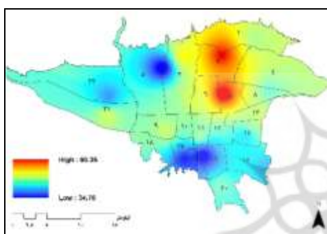
شکل ۷. وضعیت غلظت آلاینده NO 2 در شهر تهران
