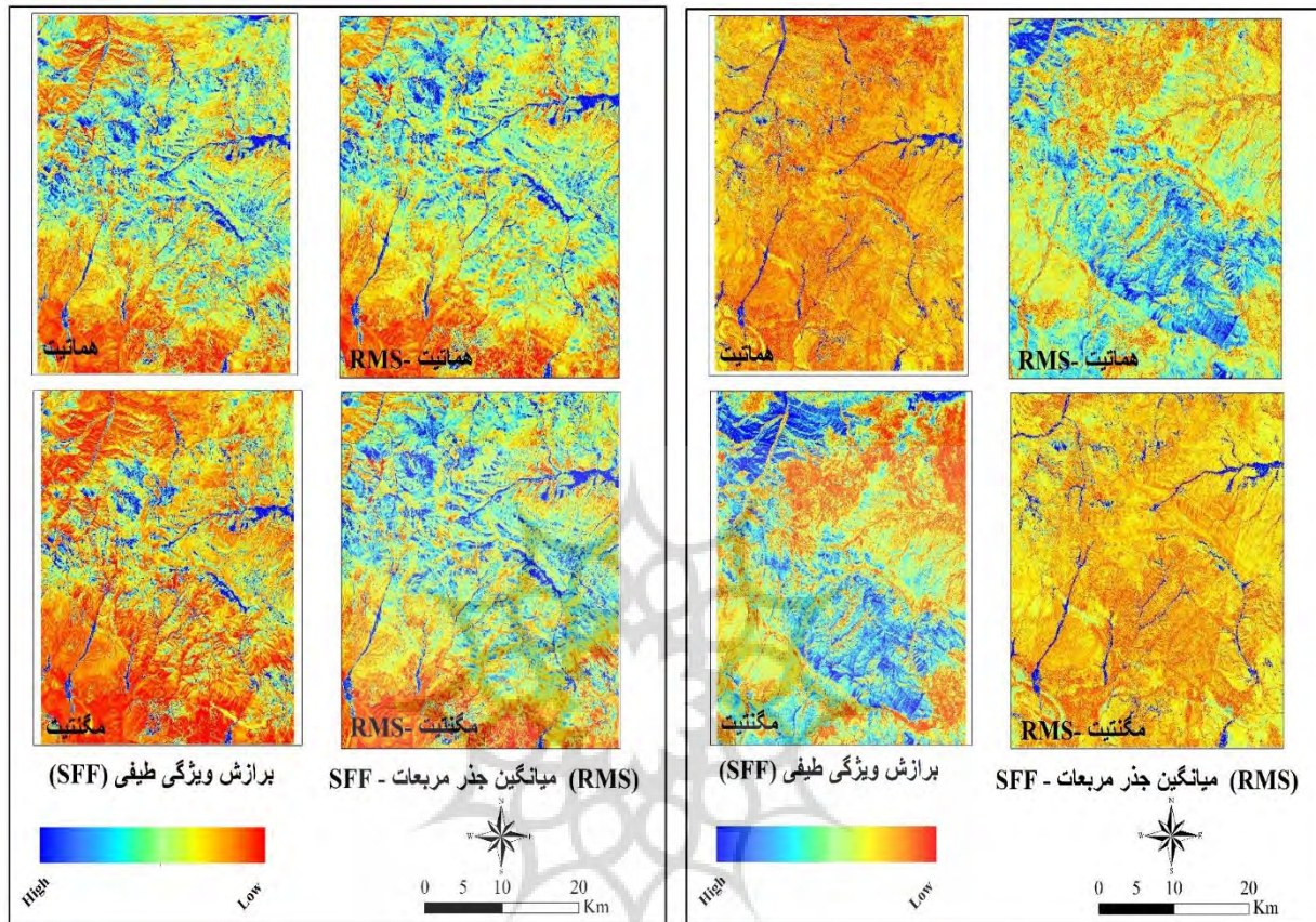
شکل ۱۰. نتایج حاصل از روش SFF (الف) بر روی داده های سنجنده
