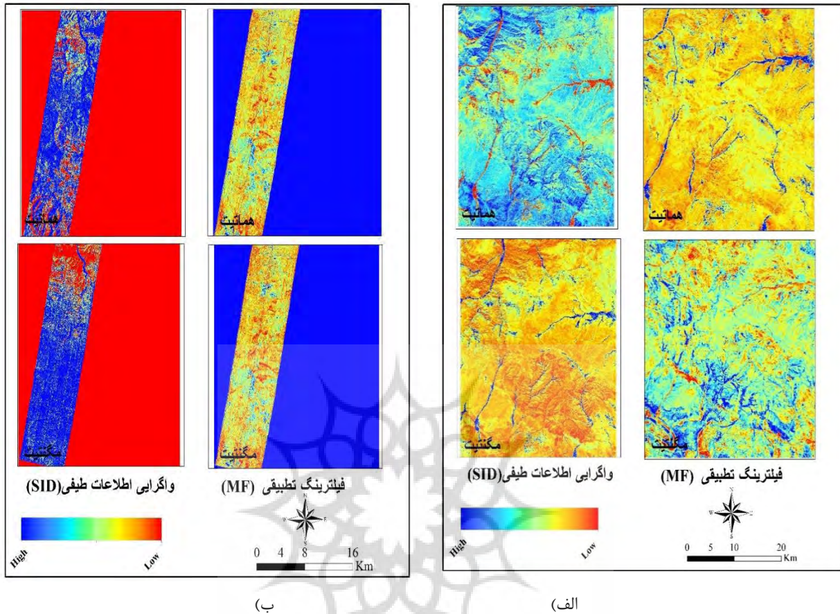
شکل ۹. نتایج حاصل از روش MF & SID الف) بر روی داده های ماهواره سنتینل ۲ و ب) داده سنجنده هایپریون
