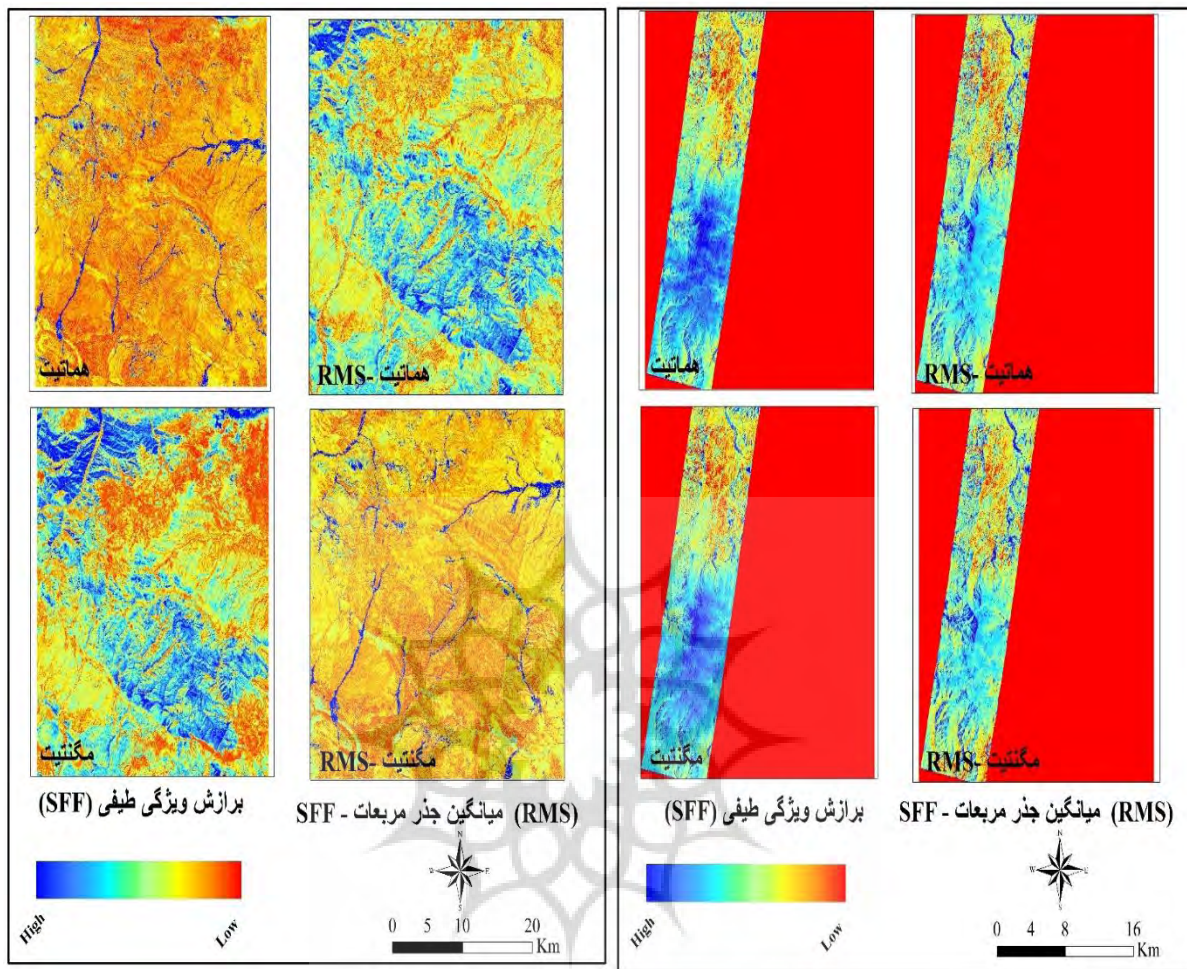
شکل ۱۱. نتایج حاصل از روش SFF (الف) بر روی داده های سنجنده هایپریون و (ب) روی داده های ماهواره سنتینل ۲
