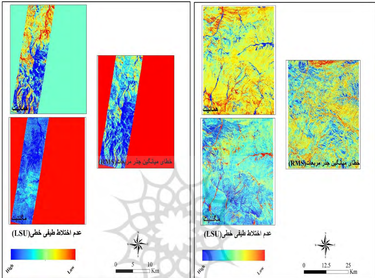
شکل ۱۳. نتایج حاصل از روش LSU الف) بر روی داده های ماهواره سنتینل ۲ و ب) بر روی داده های سنجنده هایپریون
