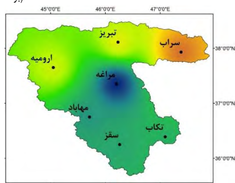
SSP1-2.6(2071-2095)
