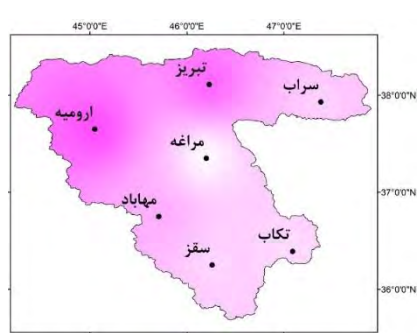
SSP1-2.6(2071-2095)
