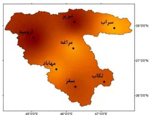
SSP5-8.5(2071-2095)
