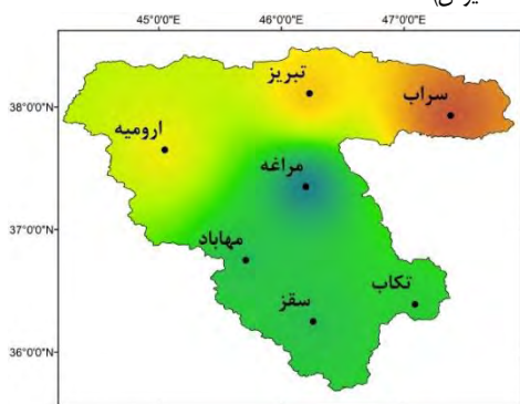
SSP1-2.6(2031-2055)
