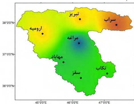
SSP5-8.5(2031-2055)
