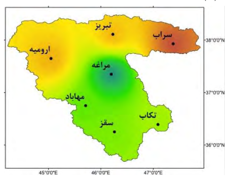
SSP5-8.5(2071-2095)
