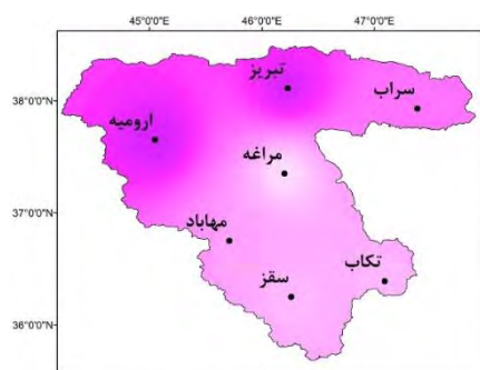
SSP1-2.6(2031-2055)
