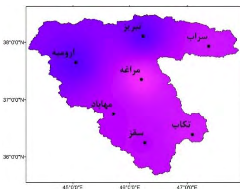
SSP5-8.5 (2031-2055)
