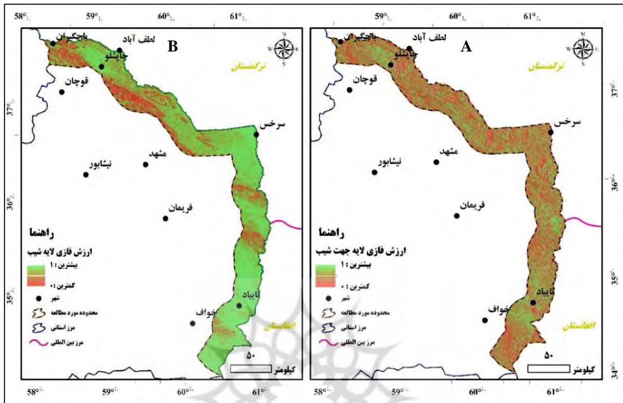
نگاره ۵: A) نقشه فازی شده جهت شیب B) نقشه فازی شده شیب
