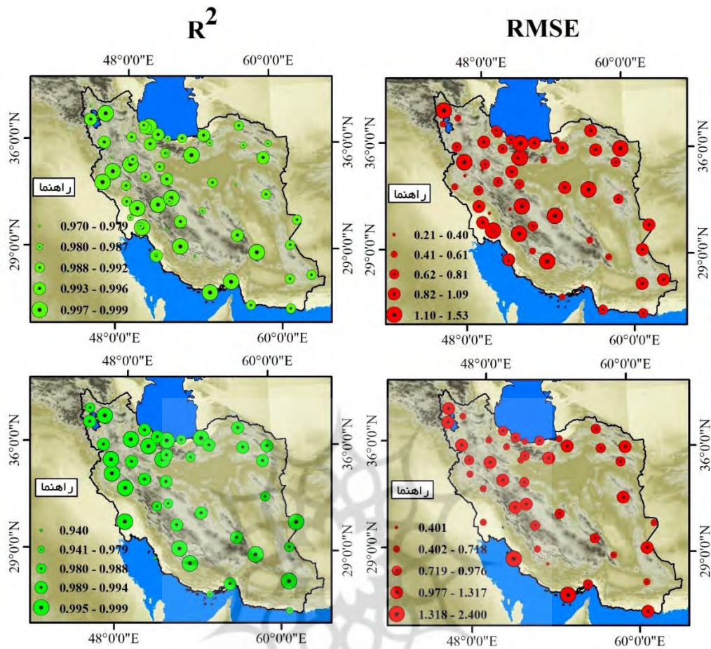
شکل ۲- سنج‌های آماری درستی سنجی دمای کمینه و بیشینه در ایران بر اساس برونداد مجموعه داده AgERA5
