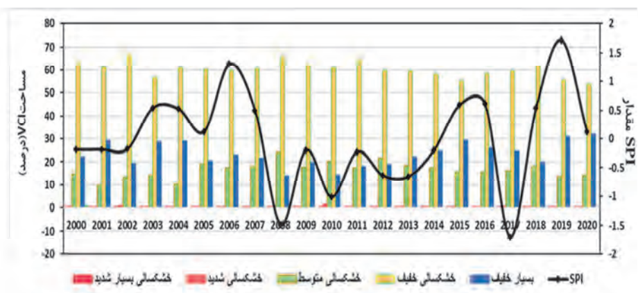
شکل ۸. تغییرات سری سالیانه شاخص SPI و طبقات گوناگون خشکسالی شاخص VCI در دوره آماری ۲۰۰۰-۲۰۲۰
