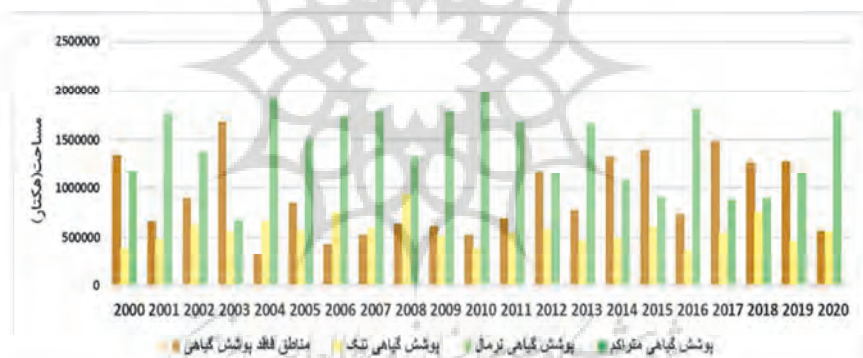
شکل ۶. تغییرات پوشش گیاهی استان لرستان براساس شاخص میانگین اختلاف نرمال‌شده پوشش گیاهی (NDVI) در دوره آماری ۲۰۰۰-۲۰۲۰
