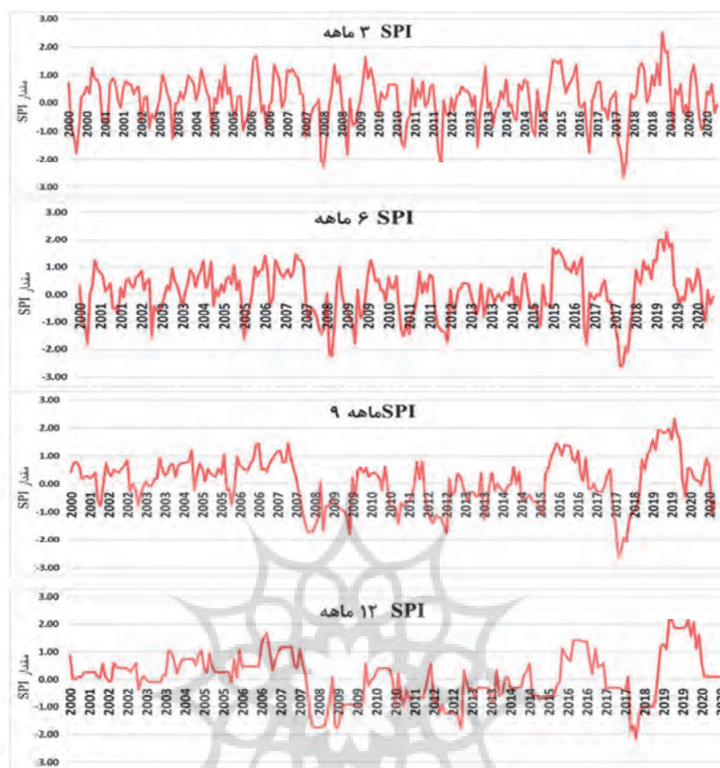
شکل ۴. تغییرات شاخص خشکسالی بارش استاندارد شده (SPI) در مقیاس‌های زمانی متفاوت سه، شش، نه و دوازده‌ماهه، طی دوره آماری ۲۰۰۰-۲۰۲۰
