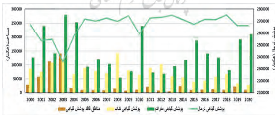
شکل ۷. تغییرات پوشش گیاهی استان لرستان براساس شاخص SAVI در دوره آماری ۲۰۰۰-۲۰۲۰
