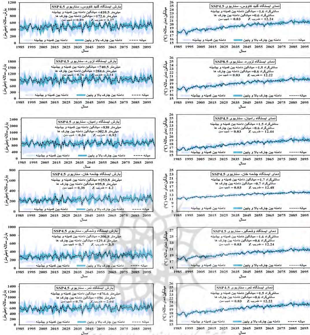
شکل ۲. روند تغییرات دما و بارش حوضه آبخیز گرگانرود تحت سناریو SSP2-4.5 طی دوره ۱۹۸۵-۲۱۰۰
