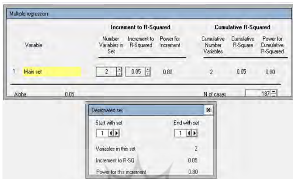
شکل ۲. خروجی برآورد حجم نمونه SPSS SAMPLE POWER
