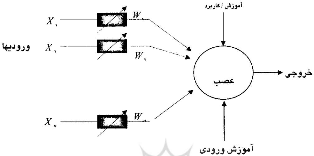
مدل ۴- عصب مک کلوج و پیترز (MCP)
