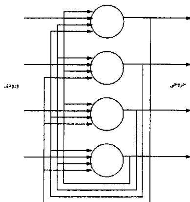
مدل ۸ - شبکه‌ی هاپل‌فید با چهار عصب
