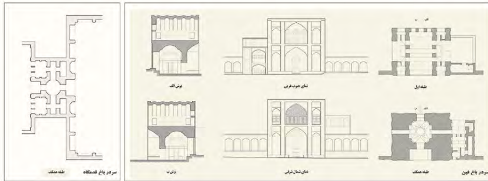
تصویر ۲۹: راست: پلان طبقات، نماها و برش‌های عمارت سردر باغ فین کاشان (جیحانی و عمرانی ۱۳۸۶، ۱۶۷)، چپ: پلان عمارت سردر باغ قدمگاه نیشابور (مرکز اسناد اداره کل میراث استان خراسان رضوی ۱۳۹۲)
