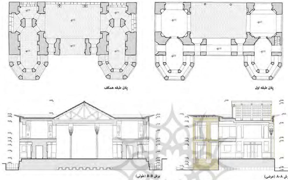
تصویر ۳۲: پلان طبقات و برش‌های طولی و عرضی کوشک اصلی (عمارت فتحعلی‌شاهی)
