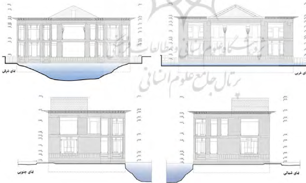
تصویر ۳۳: نماهای جوانب غربی، شرقی، شمالی و جنوبی کوشک اصلی (عمارت فتحعلی‌شاهی)
