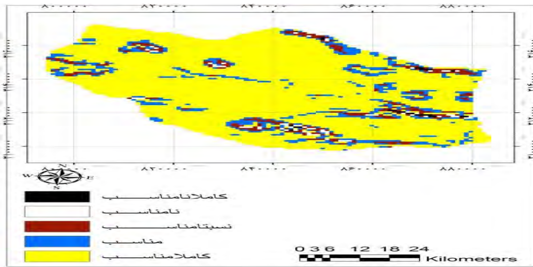
شکل ۴. لایه شیب
