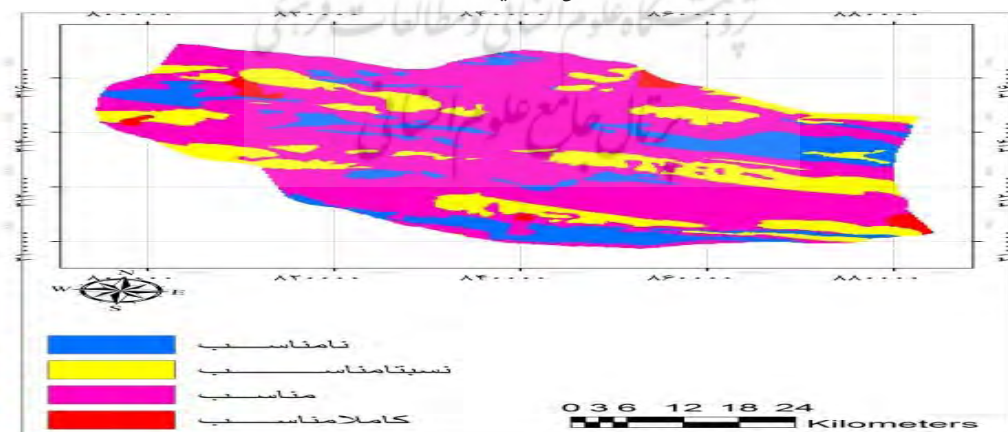
شکل ۶. لایه زمین‌شناسی
