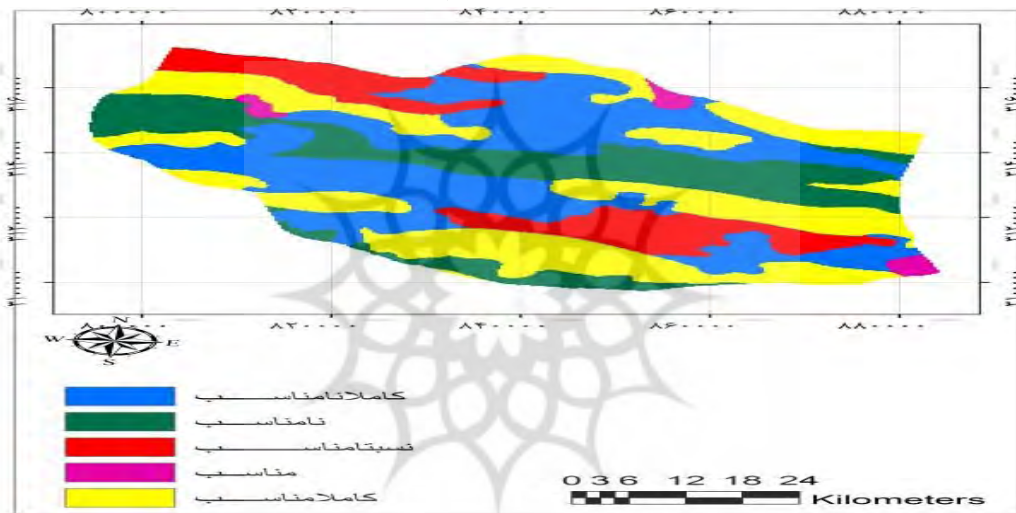
شکل ۵. لایه خاک
