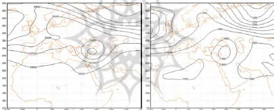
شکل (۱۷) فشار تراز ۸۵۰ میلی‌باری در روز ۷ نوامبر ۱۹۹۴ شکل (۱۸) فشار تراز ۵۰۰ میلی‌باری در روز ۷ نوامبر ۱۹۹۴
