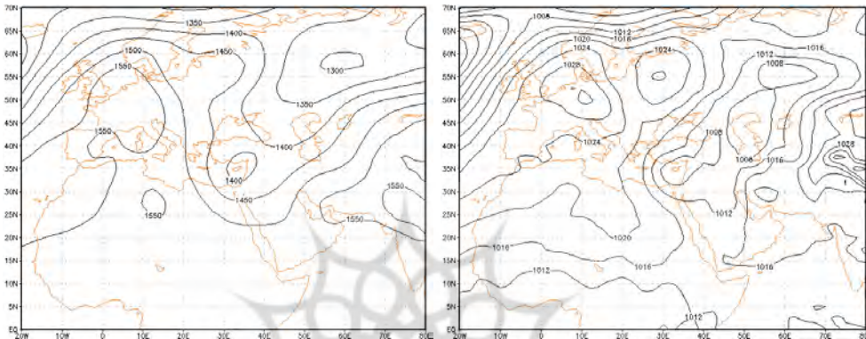
شکل (۲) فشار تراز ۸۵۰ میلیباری در روز ۲۳ دسامبر ۱۹۸۷
