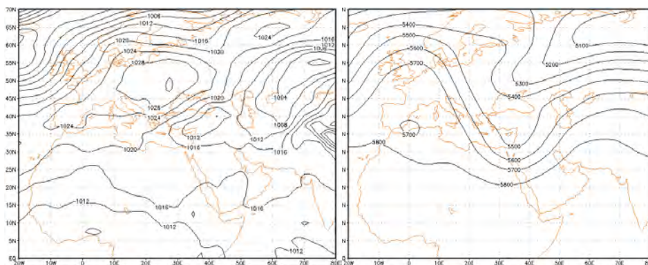
شکل (۳) فشار تراز ۵۰۰ میلیباری در روز ۲۳ دسامبر ۱۹۸۷ شکل (۴) فشار تراز دریا در روز ۲۴ دسامبر ۱۹۸۷
