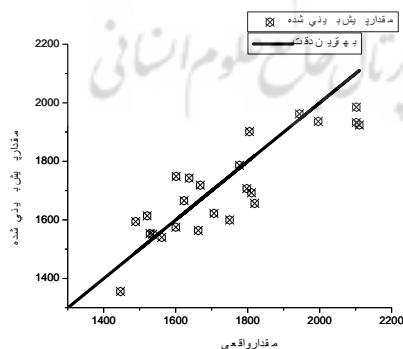
نمودار ۴: دقت پیش‌بینی در بخش صنعت
