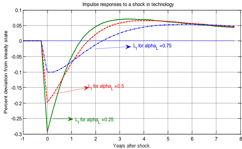
نمودار ۳: پاسخ متغیر فراغت به تکانه تکنولوژی با مقداردهی \alpha_C = \phi_L = \phi_C = 0.5 با متفاوت \alpha_L = 0.25, 0.5, 0.75
